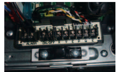
Terminal PARO/MARCHA
